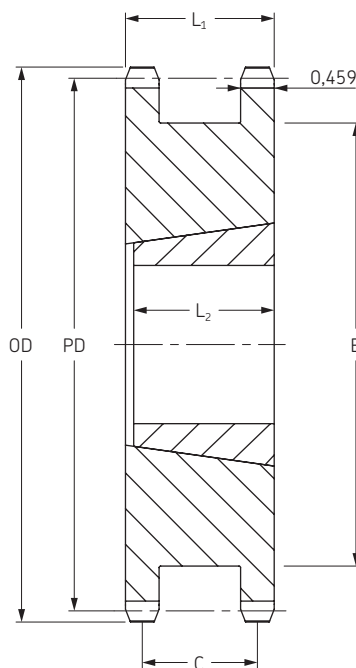
Tipo A para casquillo cónico
