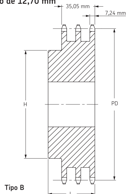
ISO 08B-3 Paso de 12,70 mm
