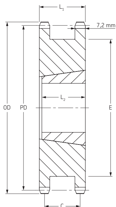
Tipo A para casquillo cónico
