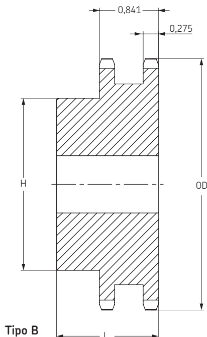
Agujero en bruto, Tipo B
