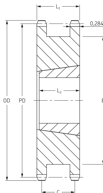
Tipo A para casquillo cónico
