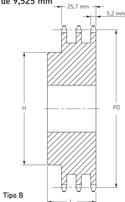
ISO 06B-3 Paso de 9,525 mm
